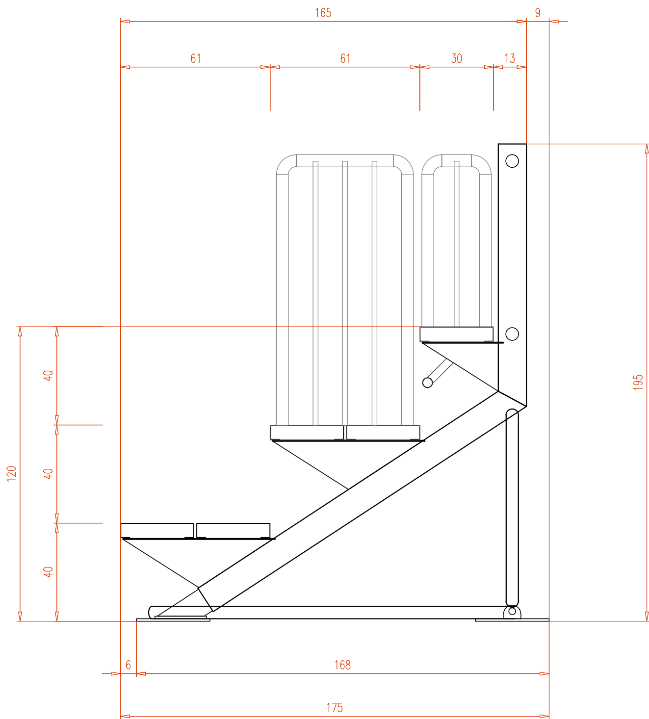
VISTA LATERALE
